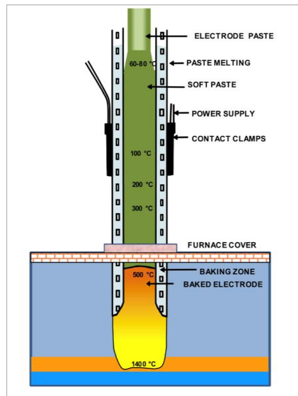
The Söderberg electrode
